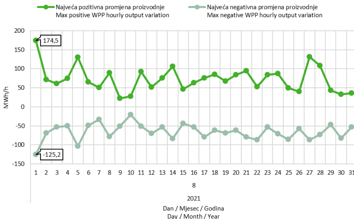
Slika 9 Maksimalna pozitivna i maksimalna negativna promjena satne proizvodnje VE u kolovozu 2021. godine
