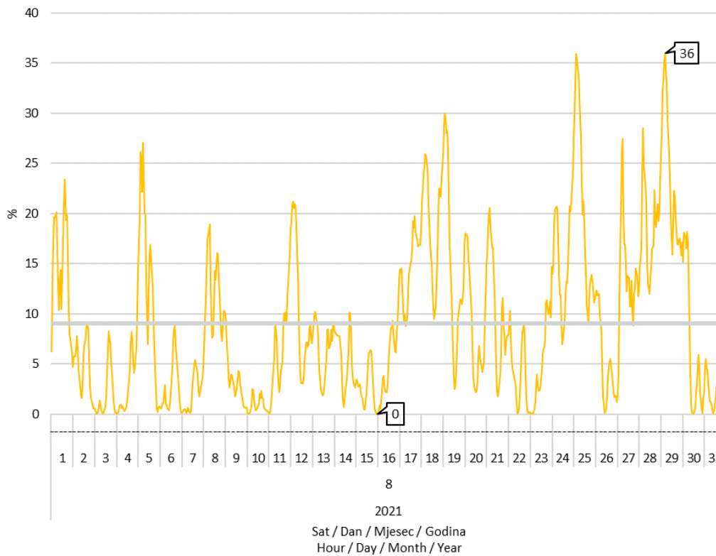
Slika 8 Udio proizvodnje vjetroelektrana u pokrivanju satnog opterećenja elektroenergetskog sustava u kolovozu 2021. godine
