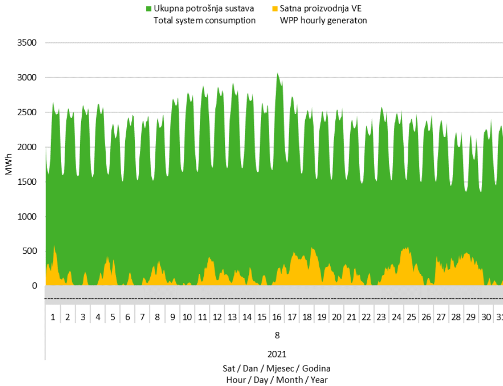
Slika 7 Usporedba satnog dijagrama opterećenja sustava i proizvodnje vjetroelektrana u kolovozu 2021. godine
