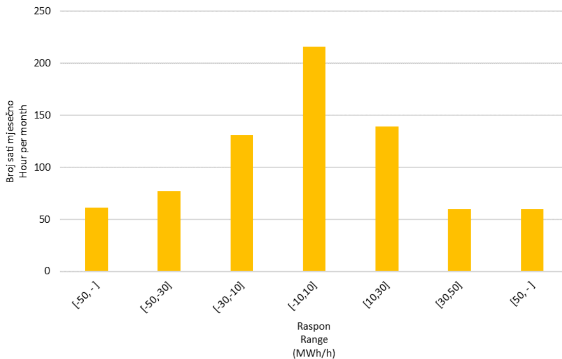
Slika 10 Statistička raspodjela satnih promjena proizvodnje VE u kolovozu 2021. godine Figure 10 Statistical distribution of WPP hourly output variations in August 2021
