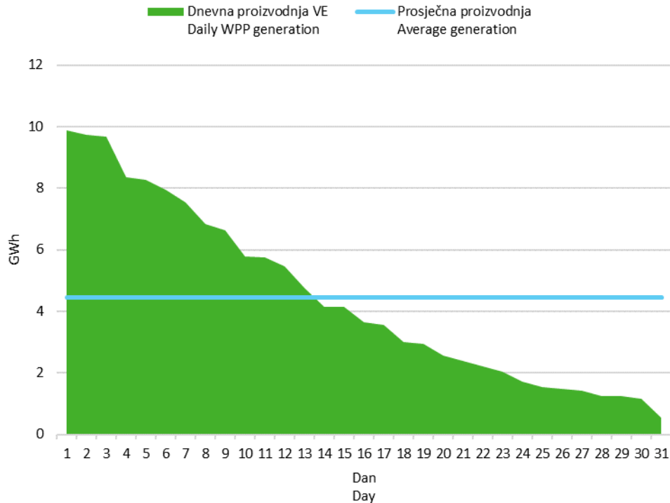
Slika 6 Krivulja trajanja dnevne proizvodnje vjetroelektrana u kolovozu 2021. godine
