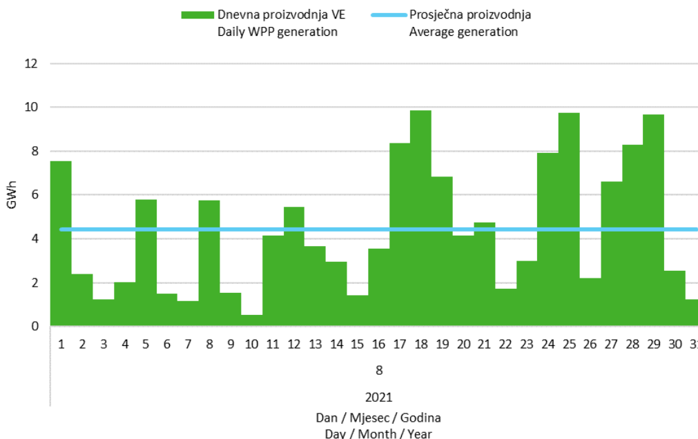
Slika 5 Dnevna proizvodnja svih vjetroelektrana u kolovozu 2021. godine Figure 5 Daily generation of all wind power plants in August 2021
