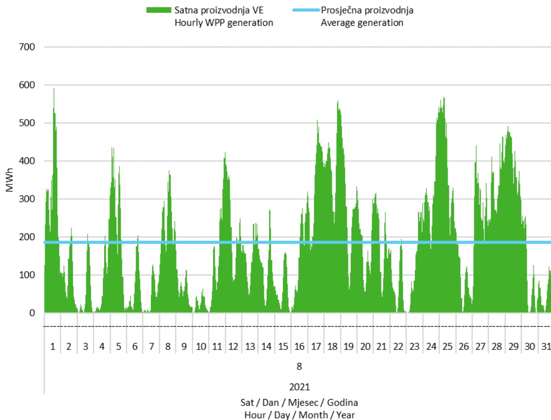
Slika 2 Satna proizvodnja svih vjetroelektrana u kolovozu 2021. godine
