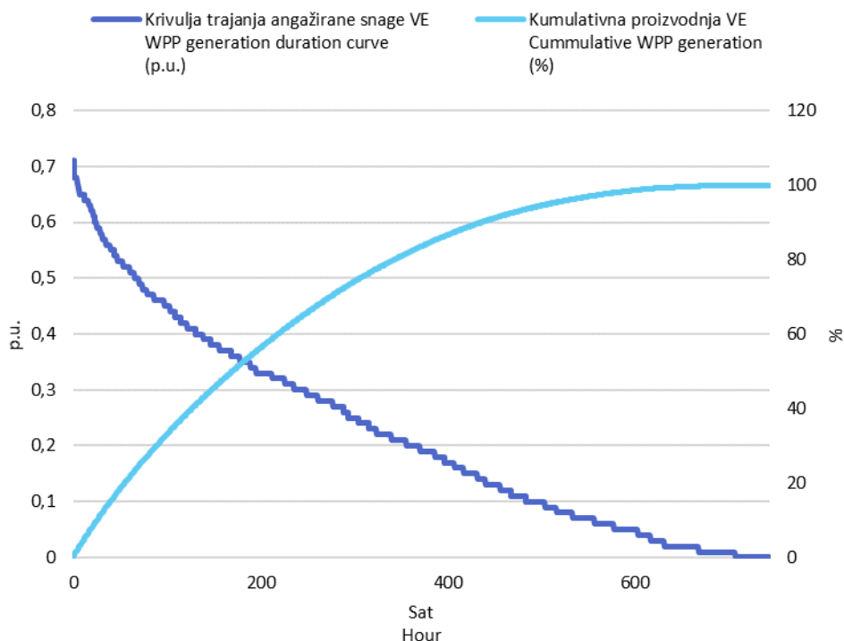
Slika 3 Krivulja trajanja angažirane snage svih VE i kumulativna proizvodnja VE u kolovozu 2021. godine u jediničnim vrijednostima
